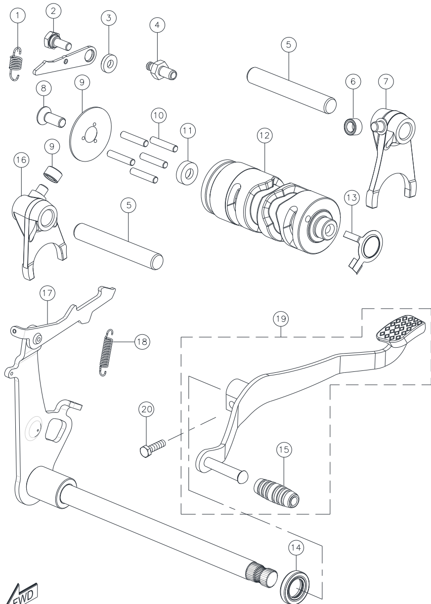
GEAR SHIFT ASSEMBLY
