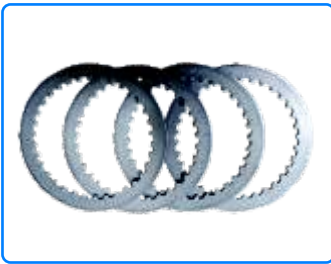
PART NO. : 520JT05075 APPLICATION : PLATE CLUTCH SUITABLE FOR : BAJAJ-XCD 135 STD. PACK : 120
